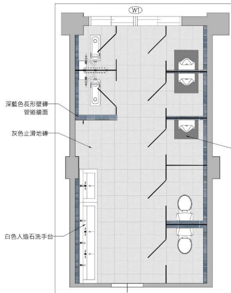
活動中心1F性別友善廁所設計平面圖
